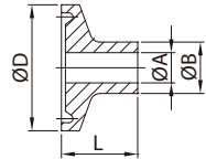
DN6~DN10 (DIN32676)
